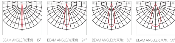
BEAM ANGLE/光束角：15° BEAM ANGLE/光束角：24° BEAM ANGLE/光束角：36° BEAM ANGLE/光束角：50°
